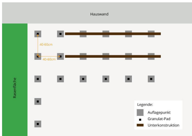
Skizze Aufbau-Unterkonstruktion
